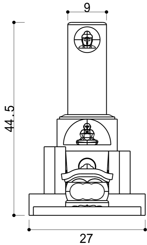
正面图
